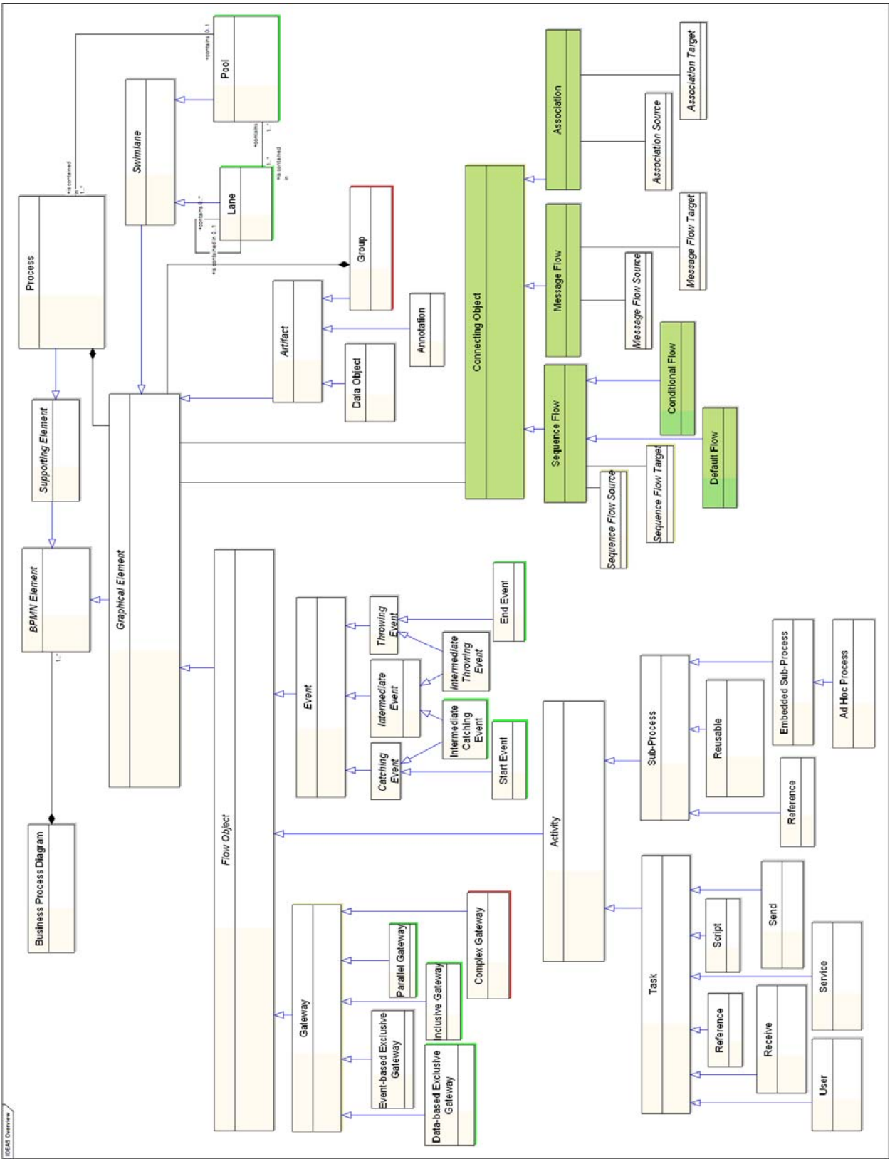
Fig. 2. BPMN 1.2 Meta-Model
